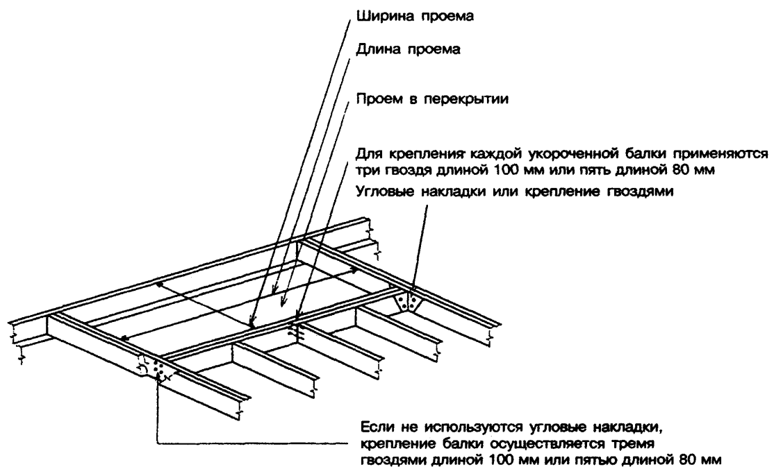
Рисунок 6-11 — Устройство консолей
