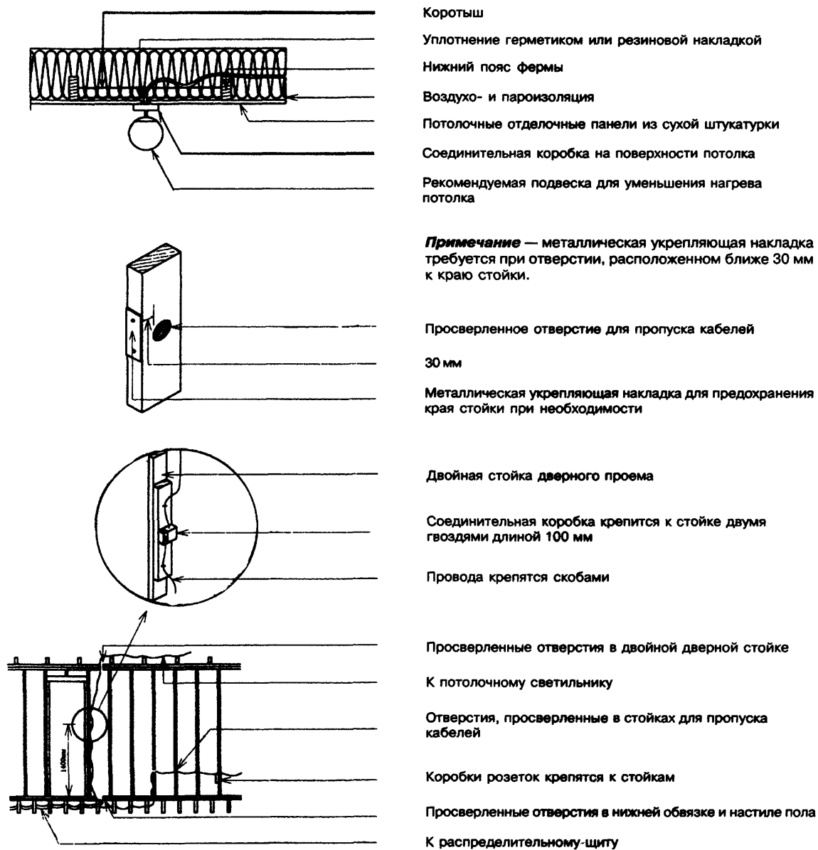
Рисунок 13-9 — Прокладка электрических проводов в элементах каркаса
