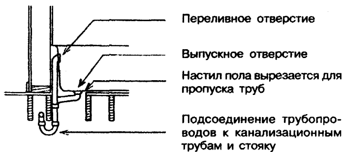
Рисунок 13-6 — Детали установки умывальника и ванны
